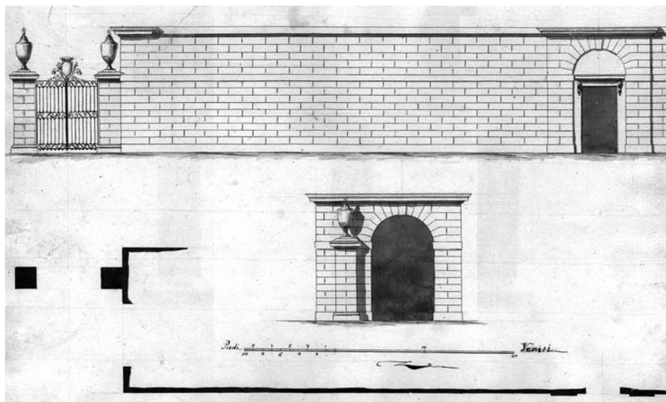
Sl.1. Nacrt glavnog reprezentativnog portala, te nadogradnje i spajanja dviju gospodarskih građevina na ulaznom pročelju agrarnog parka obitelji Garagnin u Trogiru. Građevine su spojene središnjim gospodarskim portalom. (Muzej grada Trogira, Fond Garagnin-Fanfogna)
