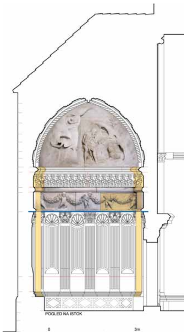
15. Unutarnji plašt istočnog zida krstionice s obilježenim intervencijama Nikole Firentinca; plava linija označava donju granicu Firentinčeve demontaže građevine (nacrt izradili: I. Valjato-Vrus – I. Tenšek; prema interpretaciji autora prilagodio: M. Košta)
