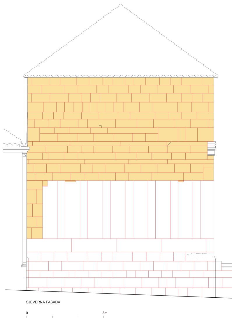
19. Vanjski plašt sjevernog zida krstionice s obilježenim intervencijama Nikole Firentinca (nacrte izradili: I. Valjato-Vrus – I. Tenšek; prema interpretaciji autora prilagodio: M. Košta)
