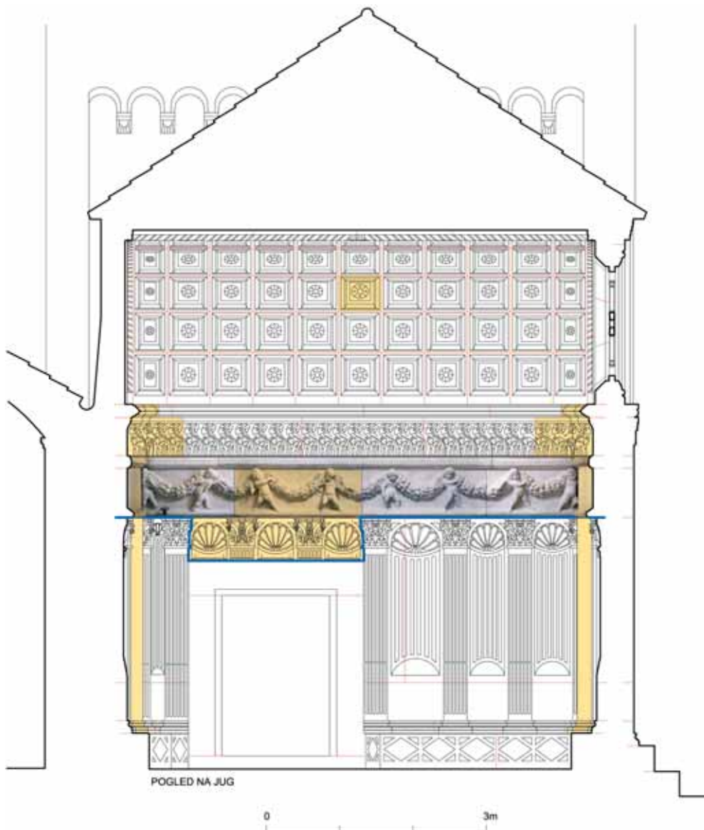
16. Unutrašnji plašt južnog zida krstionice s obilježenim intervencijama Nikole Firentinca; plava linija označava donju granicu Firentinčeve demontaže građevine (nacrte izradili: I. Valjato-Vrus – I. Tenšek; prema interpretaciji autora prilagodio: M. Košta)
