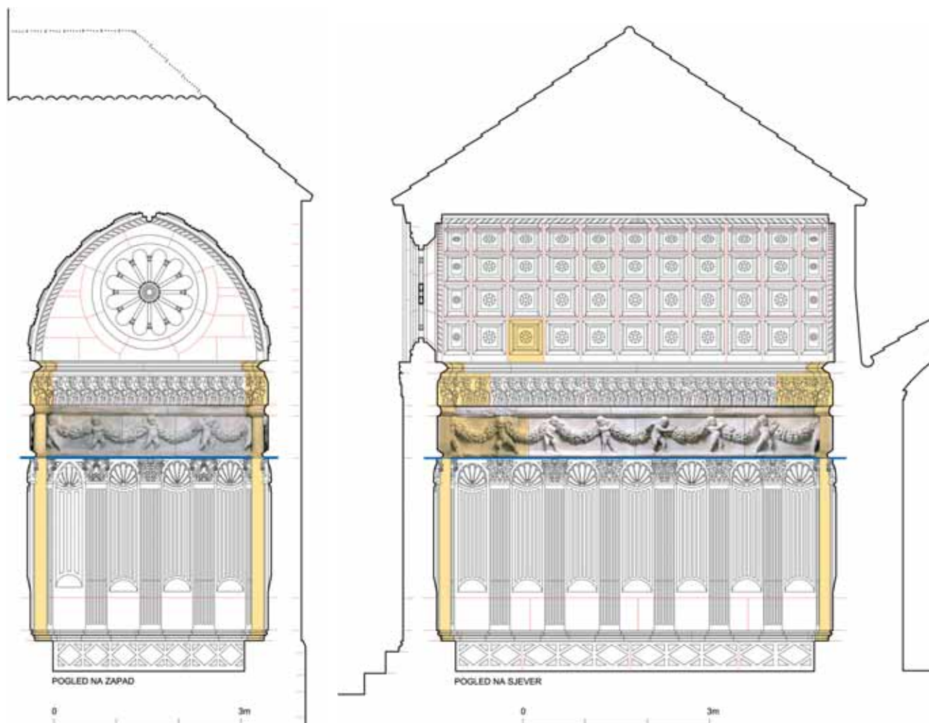
17. Unutarnji plašt zapadnog zida krstionice s obilježenim intervencijama Nikole Firentinca; plava linija označava donju granicu Firentinčeve demontaže građevine (nacрте izradili: I. Valjato-Vrus – I. Tenšek); prema interpretaciji autora prilagodio: M. Košta)
