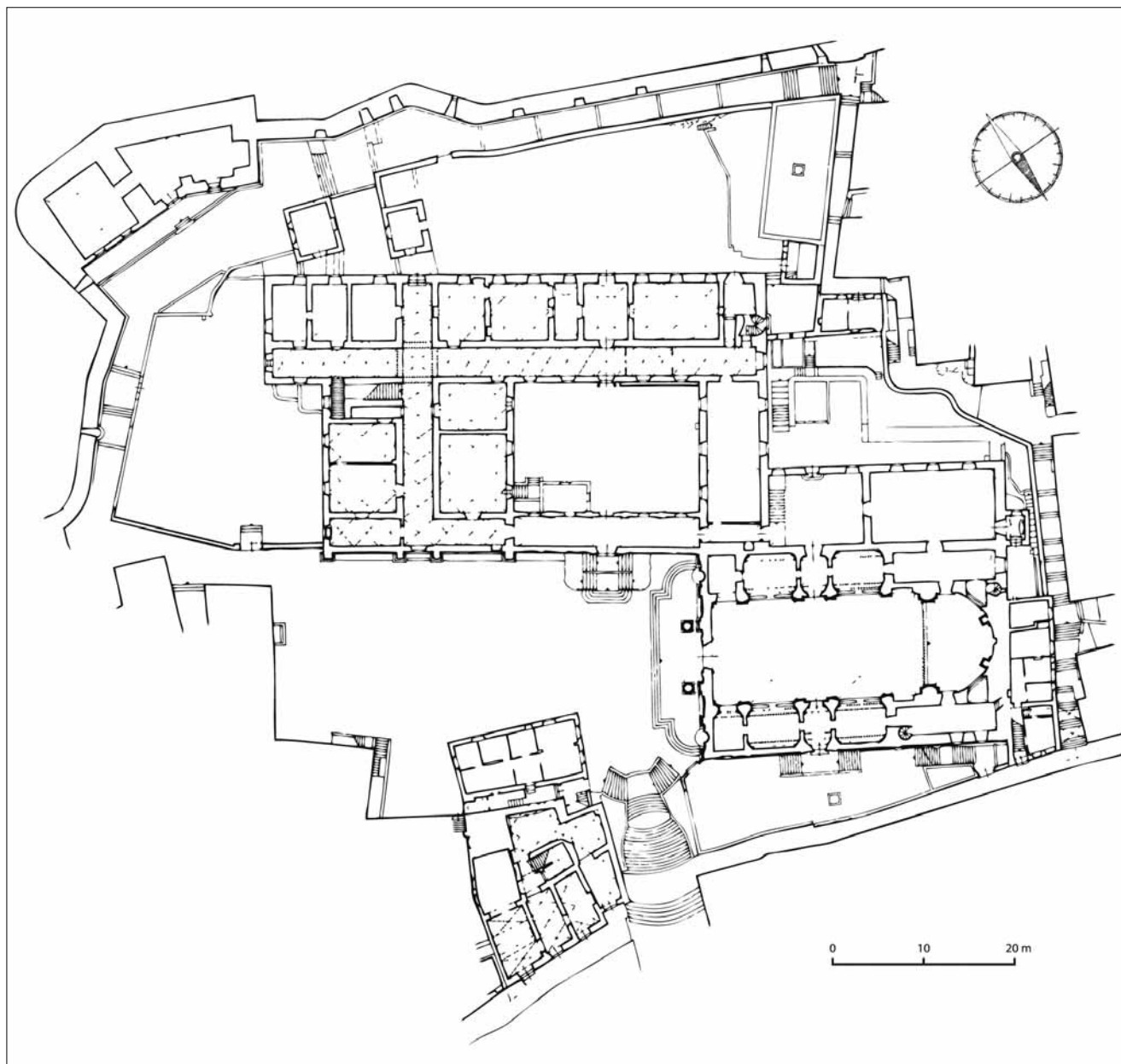
10 Isusovačka crkva i kolegij u Dubrovniku, sadašnje stanje (grafička obrada: T. Pugelnik) Jesuit church and college in Dubrovnik, current
