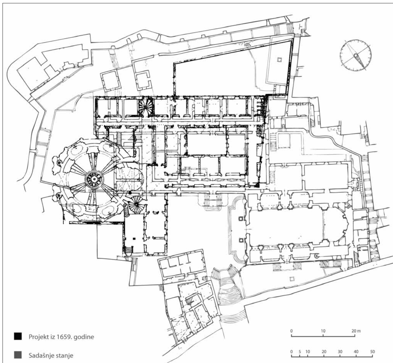
8 Prikaz planiranog smještaja isusovačkoga sklopa prema projektu iz 1659. godine (skala u metrima i dubrovačkim laktima; grafička obrada: T. Pugelnik)
