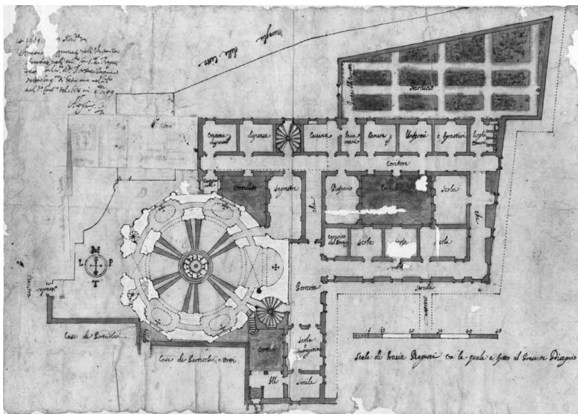
6 Serafino Fabrini, projekt za isusovačku crkvu i kolegij u Dubrovniku, 1659. (prikaz s objektima namijenjenima rušenju)
