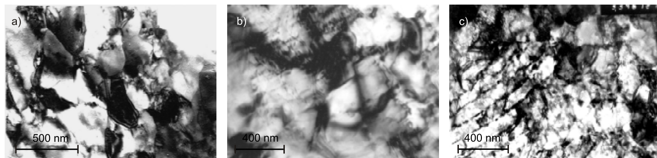
Figure 6. Structure of low carbon steels after warm ECA pressing: a - 0,17 % C - steel; b - 0,21 % C - 0,89 % Mn - 0,78 % Si - 0,16 % V - steel; c - 0,23 % C - 1,24 % Mn - 0,75 % Si - steel; a - ECAP; T_{def} = 500 °C; b - c - ECAP; T_{def} = 550 °C
