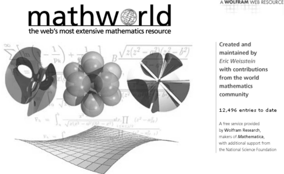
Slika 1. MathWorld
