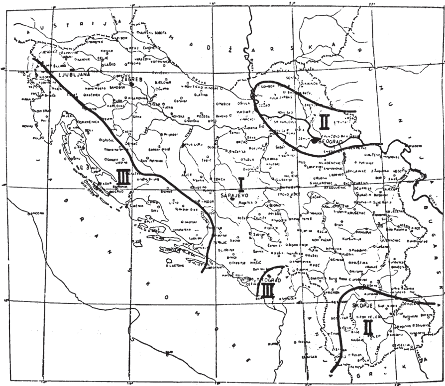
Slika 2. Podjela teritorija Jugoslavije na geografske zone brzine vjetra, prilog Pravilniku o tehničkim propisima o djelovanju vjetra na noseće čelične konstrukcije (1964.). Izvor: B. FURUNDŽIĆ, S. FURUNDŽIĆ, Zbirka tehničkih propisa , knj. 1, 596.
