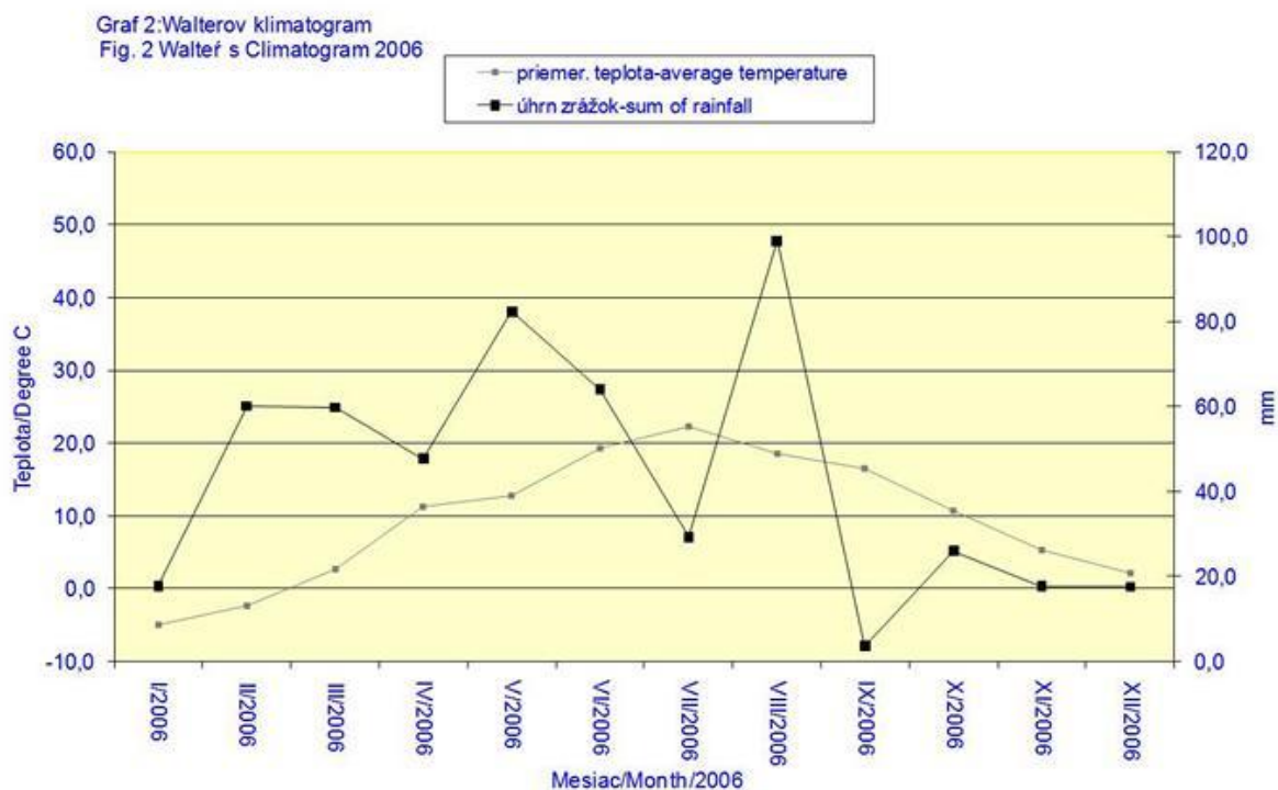
Figure 2. Walter's Climatogram 2006 Obrázok 2. Walterov klimatogram 2006
