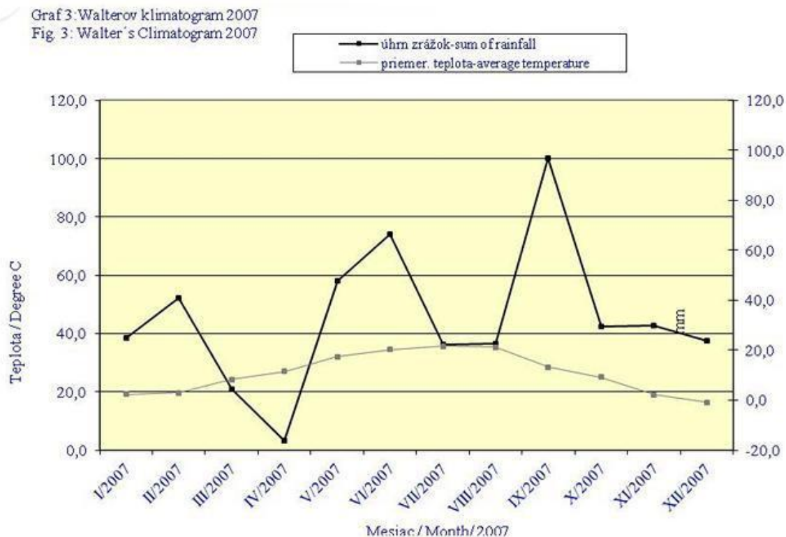
Figure 3. Walter's Climatogram 2007 Obrázok 3. Walterov klimatogram 2007
