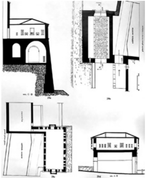
Sl. 12 – Presjeci Novih vrata 83
